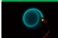
らせん状の美しいビーム
